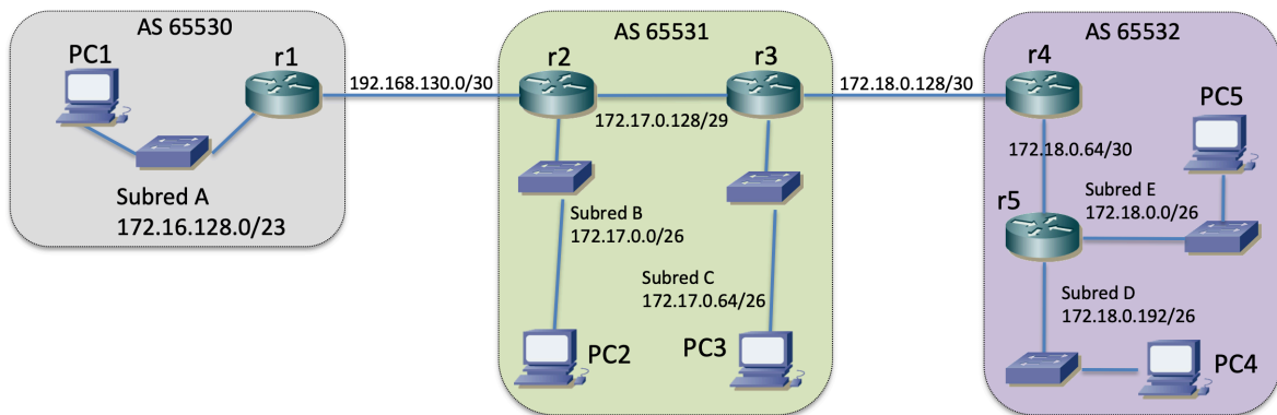
Figura 3 - iBGP en sistema de tránsito
