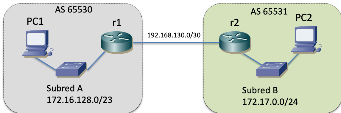
Figura 1 - Topología básica eBGP
