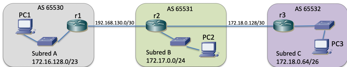
Figura 2 - Topología con 3 ASs
