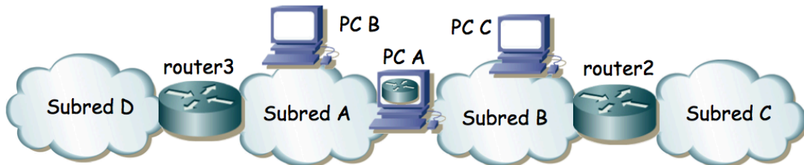
Figura 2 - Topología para prueba de interoperabilidad
