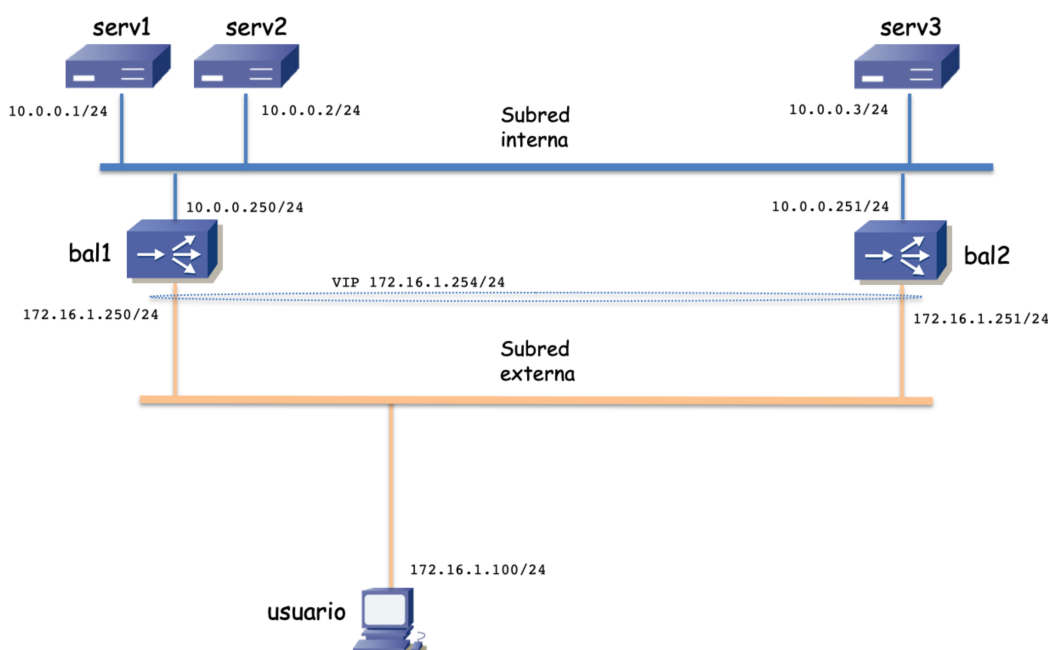
Figura 1 - Topología capa 3
