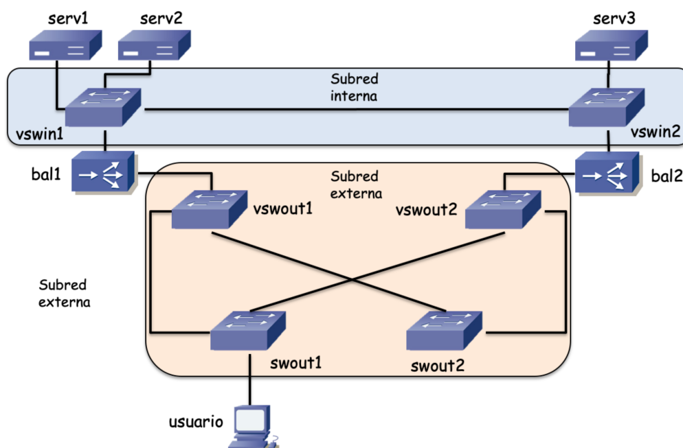
Figura 2 - Topología Ethernet
