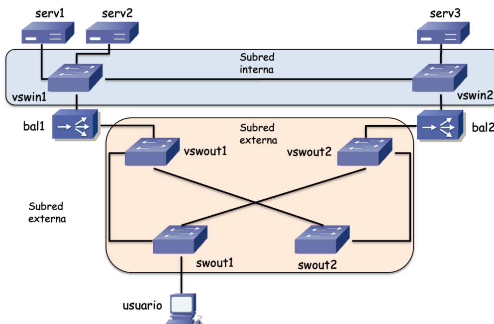
Figura 2 - Topología Ethernet
