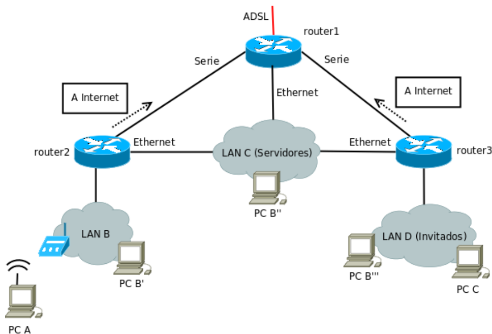
Figura 1.- Topología de red a construir
