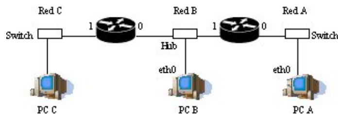
Figura 4.- 2 routers conectando 4 redes
