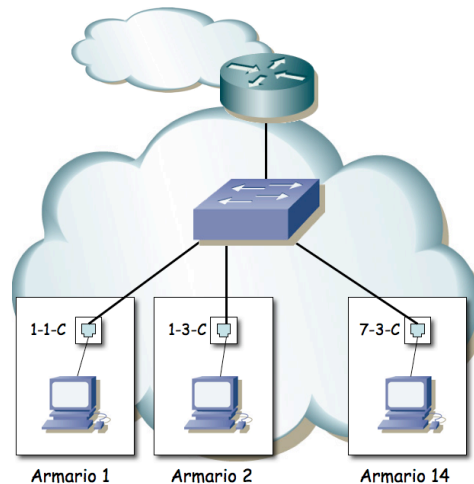
Figura 4.- LAN de prácticas
