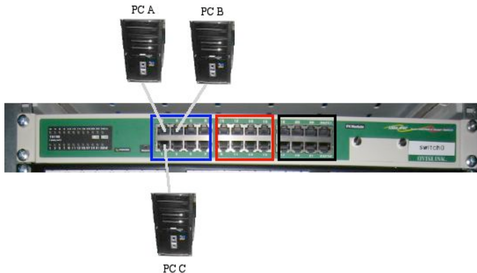
Figura 2.- Conexión de PCs a switch
