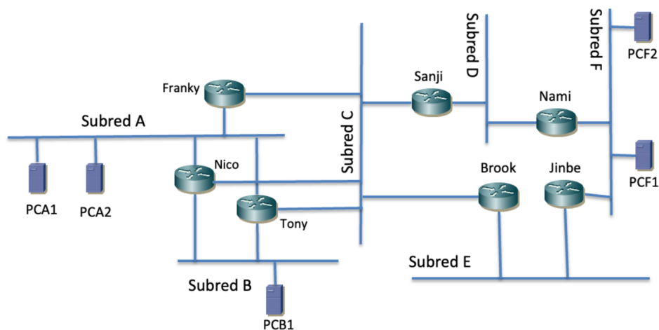
Figura 82 – Topología de capa 3 para la cuestión (d)
