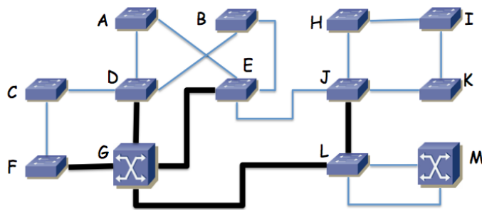
Figura 16 – Topología física
