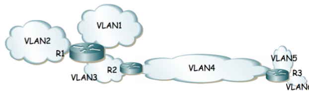
Figura 32 - Topología de nivel IP
