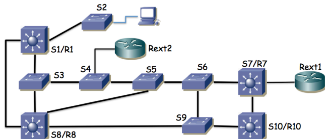
Figura 12.- Topología física
