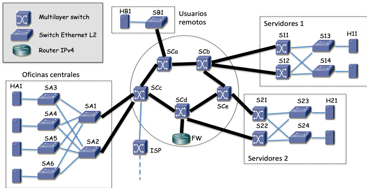
Figura 60 – Topología física
