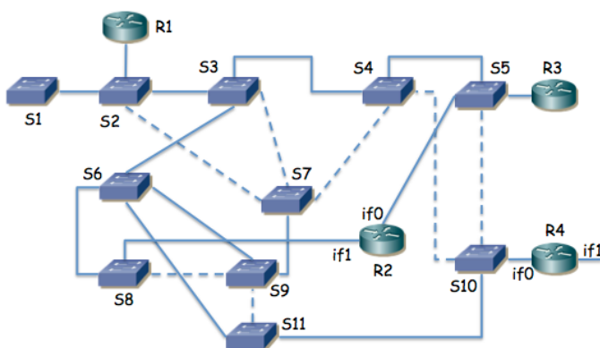
Figura 2.- Topología física/enlace
