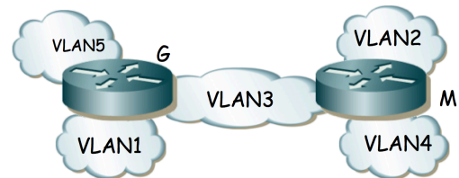
Figura 17 – Topología de nivel de red
