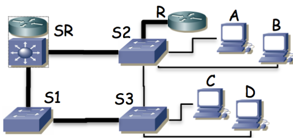
Figura 21 - Topología física
