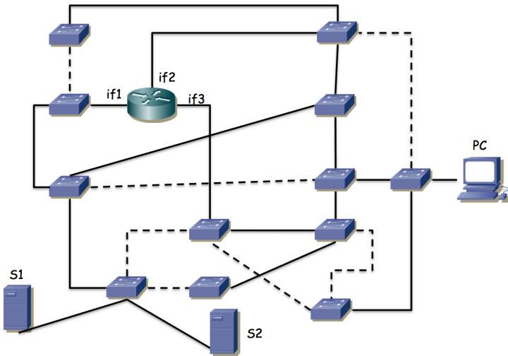
Figura 19.- Topología física/enlace
