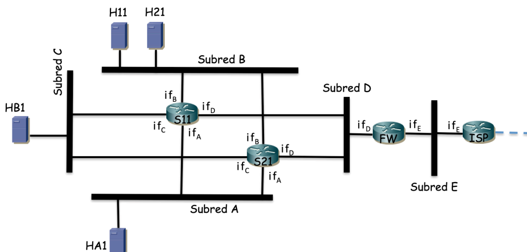
Figura 62 – Topología capa 3
