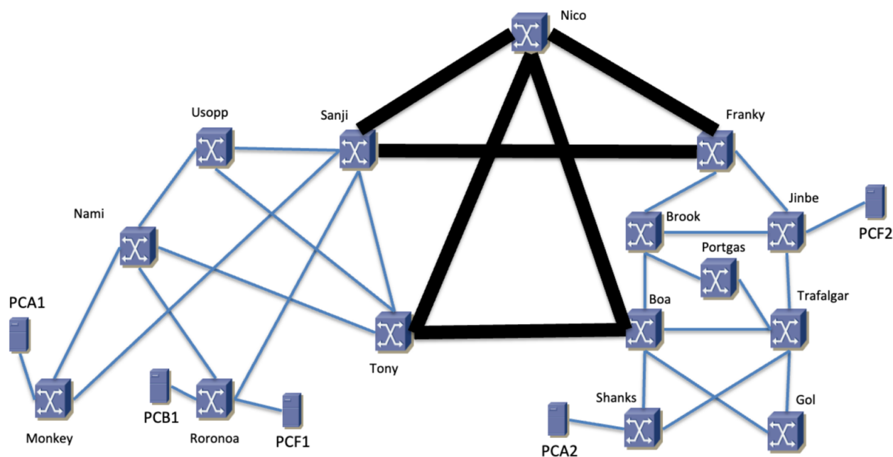
Figura 80 – Topología física
