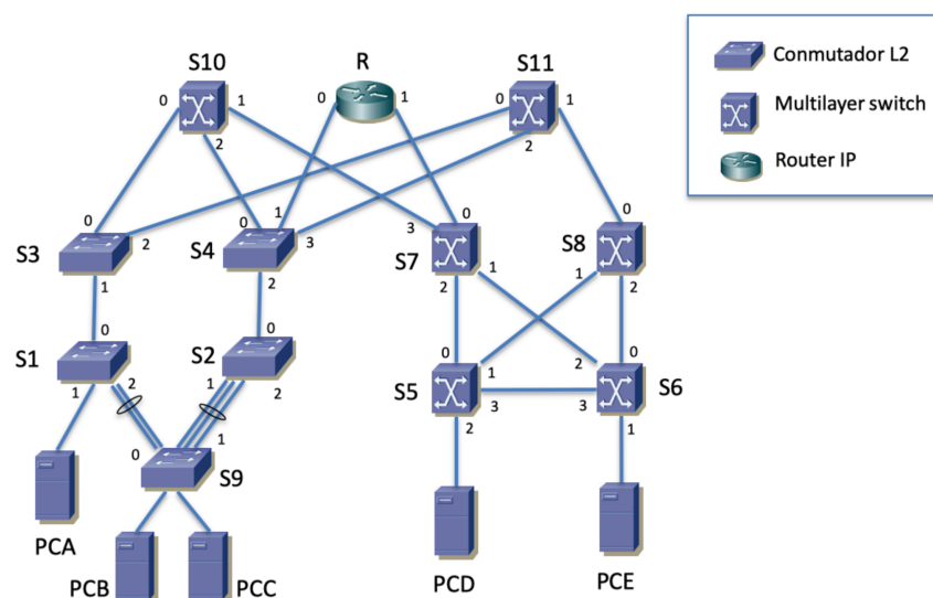
Figura 70 – Topología física
