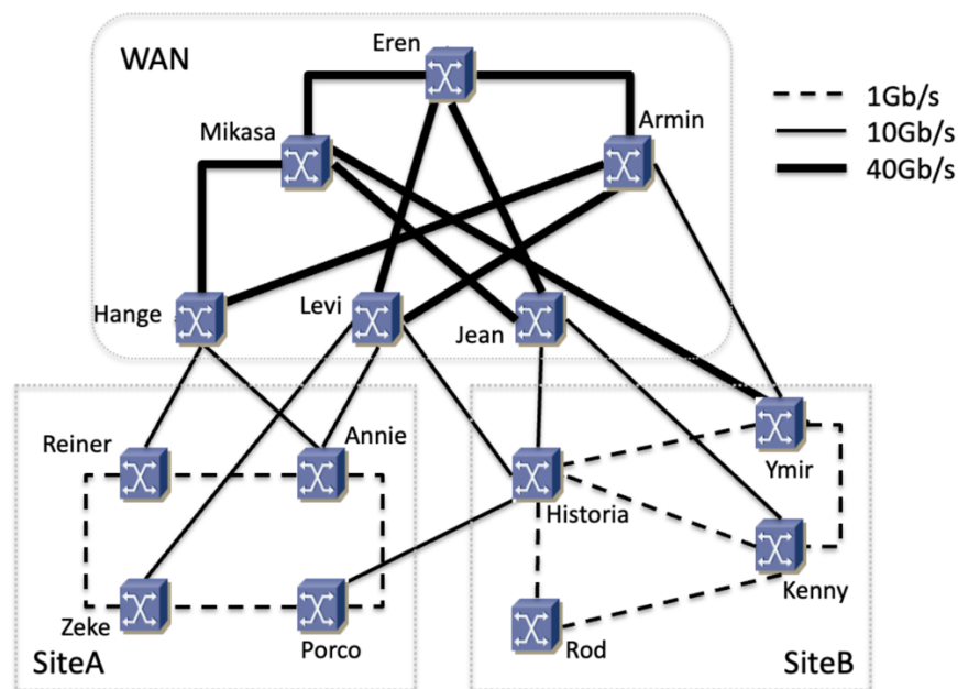
Figura 83 – Topología física
