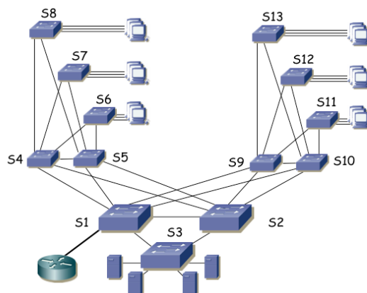
Figura 11.- Topología física
