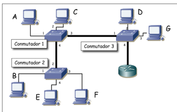
Figura 24.- Topología física
