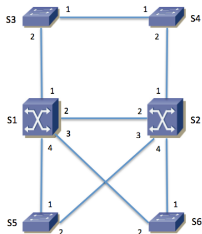
Figura 39 – Topología física
