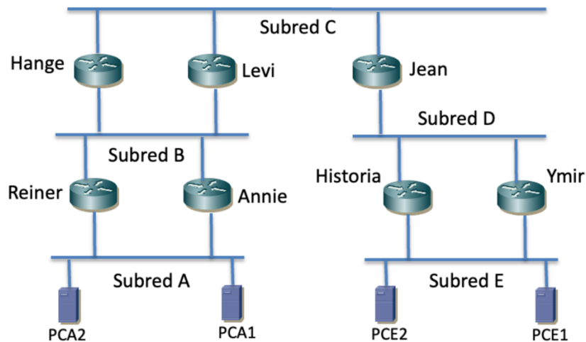
Figura 85 – Topología de capa 3 para la cuestión (d)
