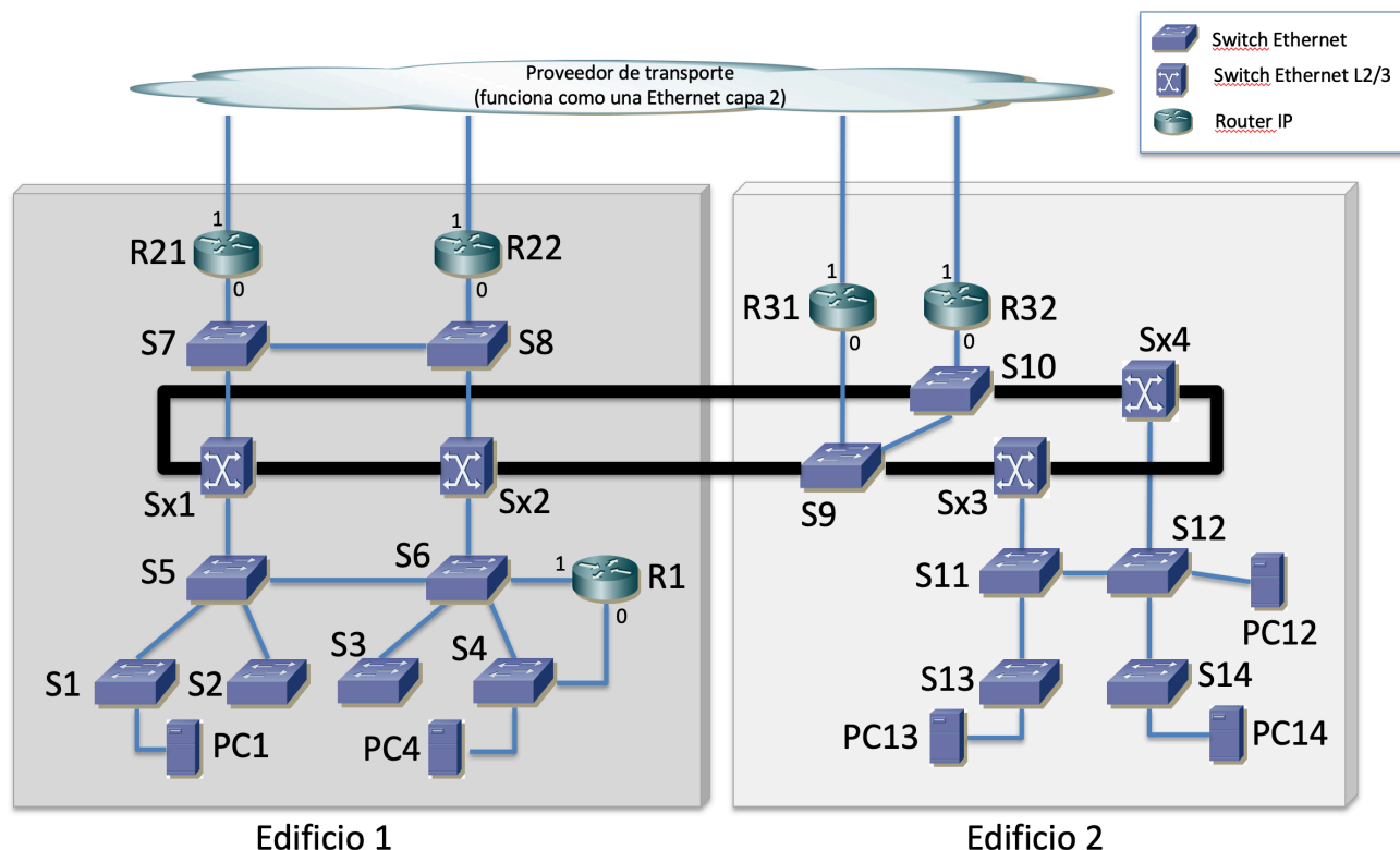
Figura 63 – Topología física
