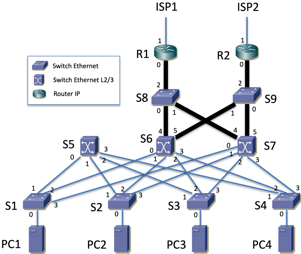
Figura 68 – Topología física
