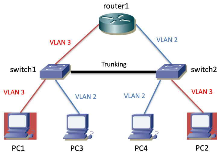
Figura 7- Topología física
