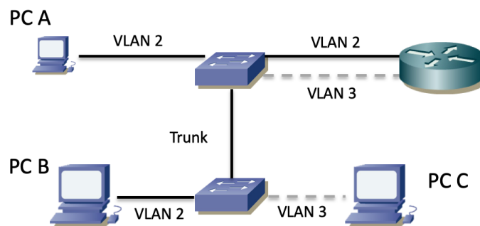
Figura 6 – Topología física empleando un enlace de trunk
