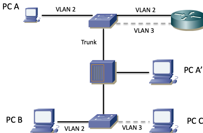
Figura 7- Un trunk con un hub interpuesto
