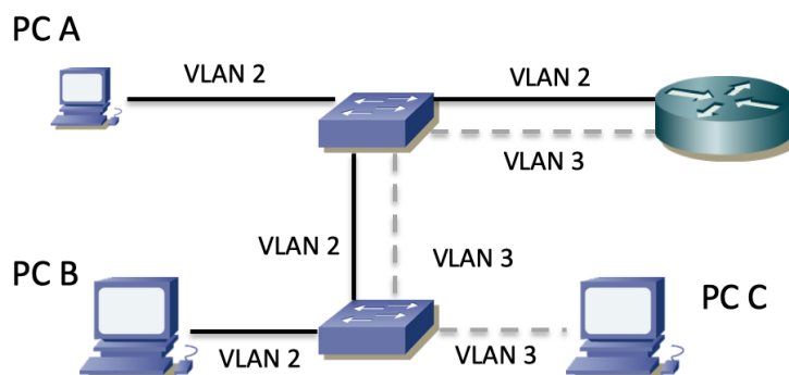
Figura 4 – Topología física con 2 switches
