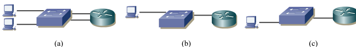
Figura 1 – Topología a) física, b) VLAN 2, c) VLAN 3
