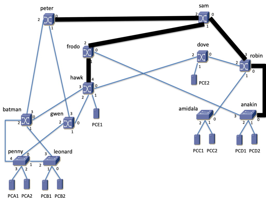
Figura 1 – Topología física
