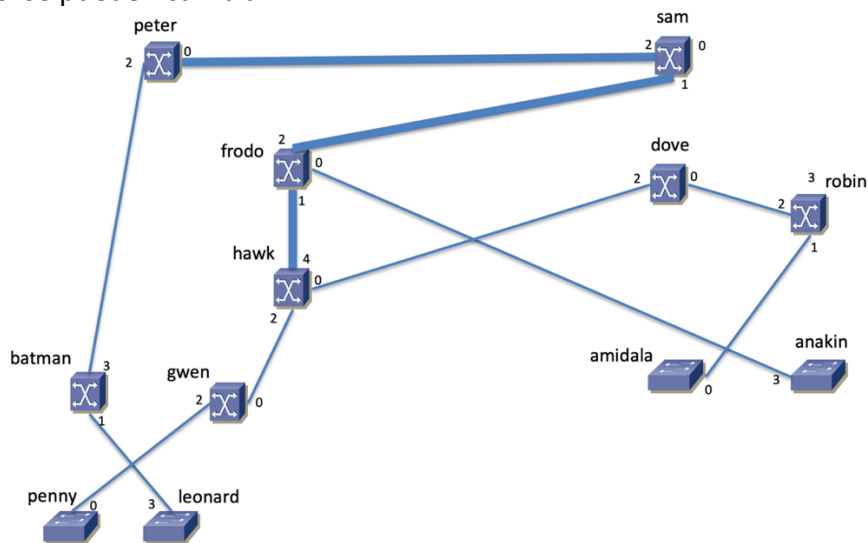
Figura 3 – Topología de respuesta a la cuestión (b)
