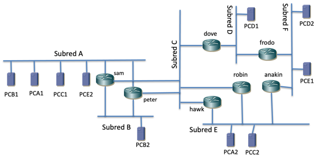
Figura 5 – Topología de capa 3 para la cuestión (d)
