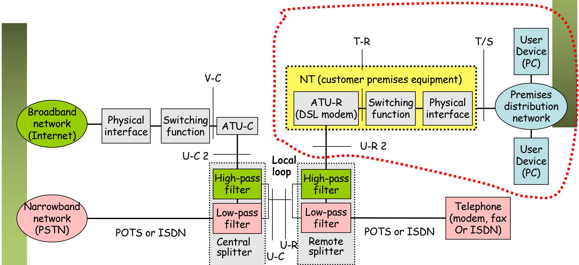
Figura 1-1/G.992.1 - Modelo de referencia del sistema ADSL
