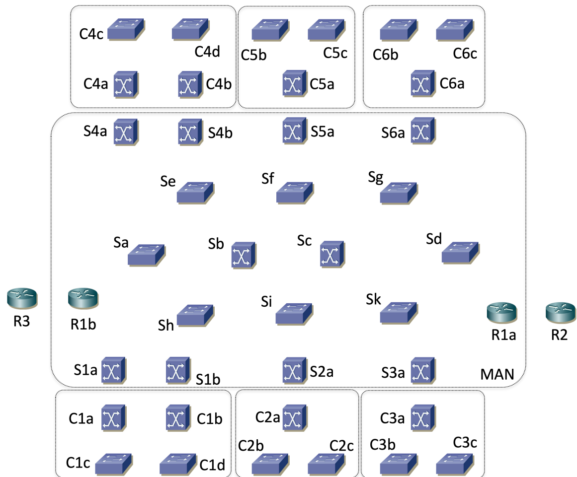
Figura 4b - Árbol de expansión resultante de la configuración para la VLAN de interconexión para la Empresa2
