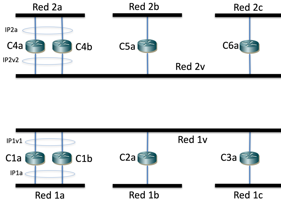
Figura 3 – Topología de nivel IP
