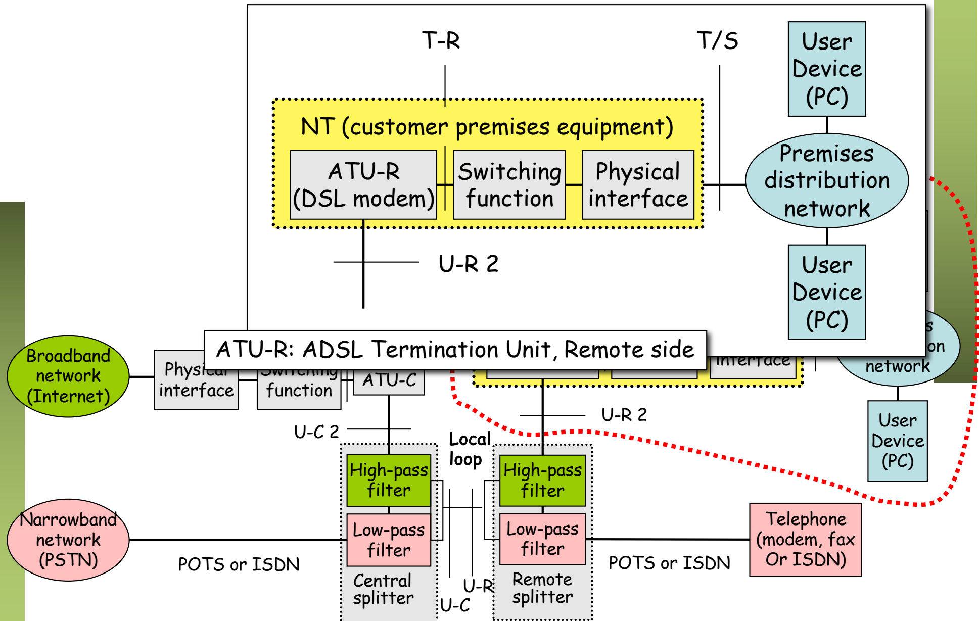
Figura 1-1/G.992.1 - Modelo de referencia del sistema ADSL
