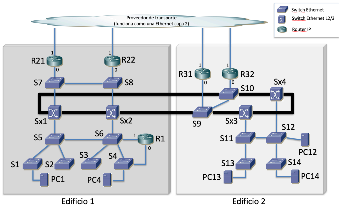
Figura 63 – Topología física
