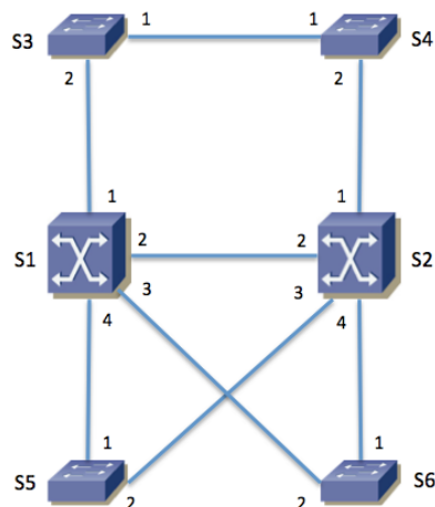
Figura 39 – Topología física
