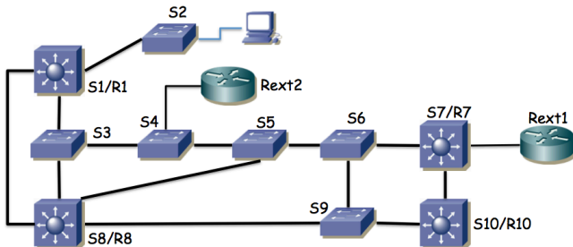
Figura 12.- Topología física
