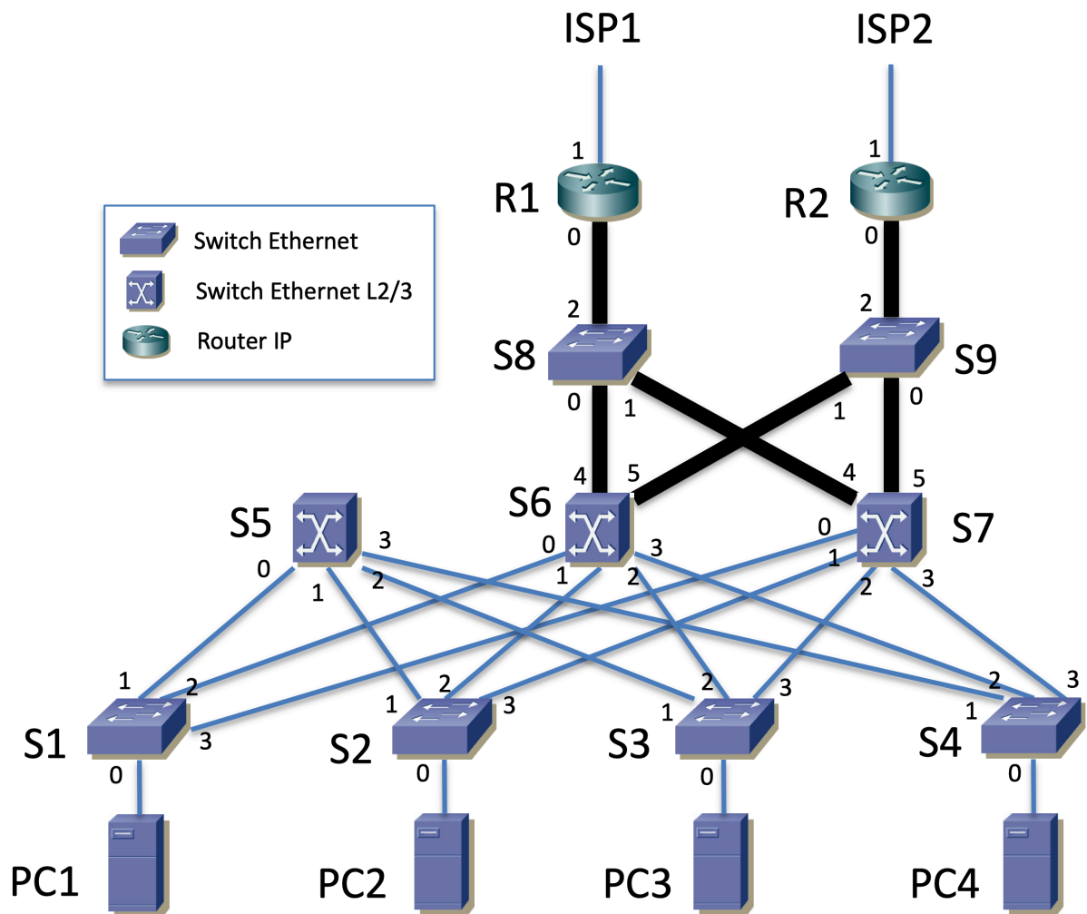
Figura 68 – Topología física
