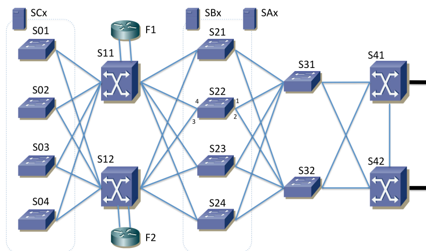
Figura 49 - Topología física
