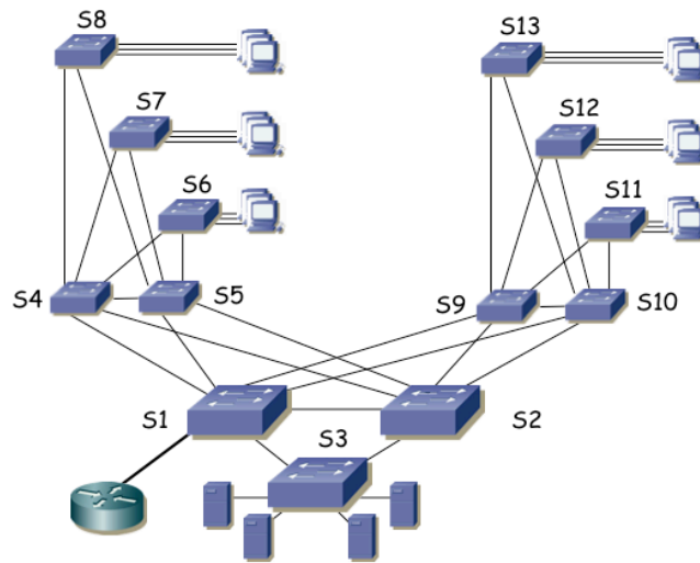
Figura 11.- Topología física
