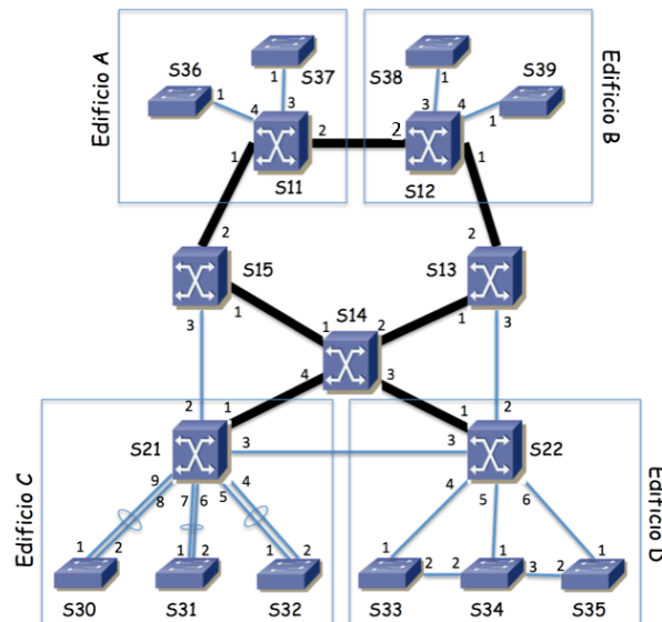
Figura 45 - Topología física
