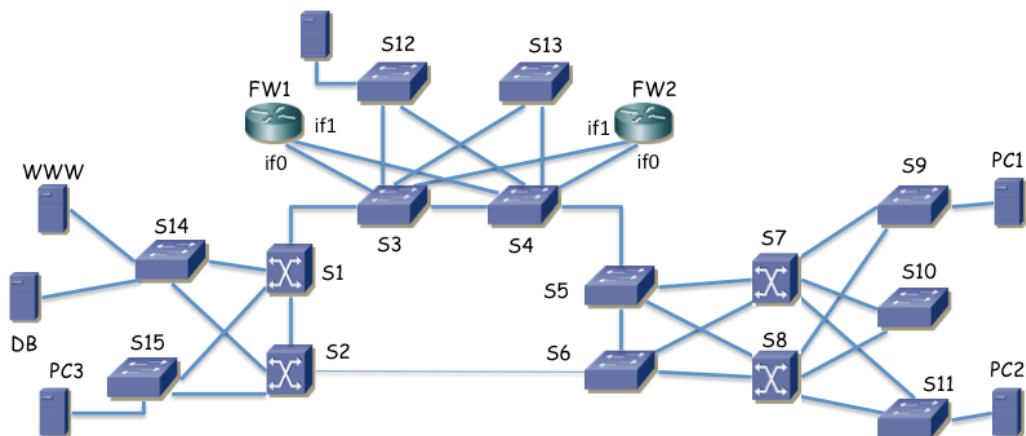
Figura 51 – Topología física
