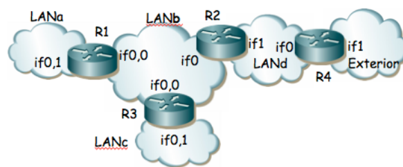
Figura 3.- Topología de nivel de red
