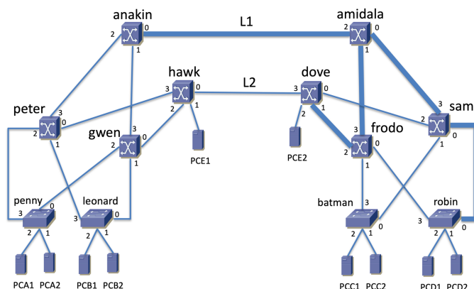
Figura 77 – Topología física
