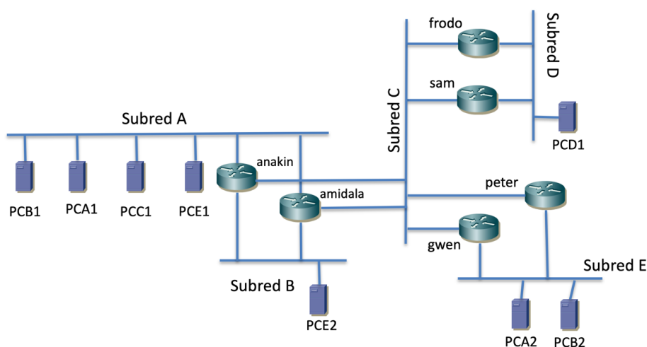
Figura 79 – Topología de capa 3 para la cuestión (d)
