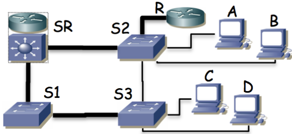
Figura 21 - Topología física
