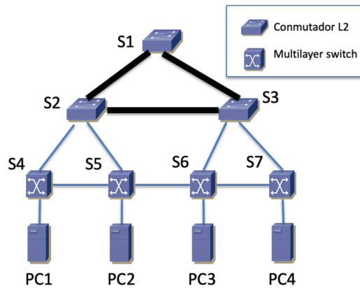
Figura 75 – Topología física
