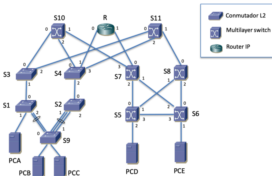
Figura 70 – Topología física
