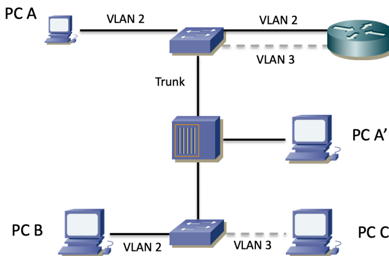
Figura 7- Un trunk con un hub interpuesto
