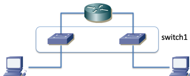
Figura 3 – Topología virtual
