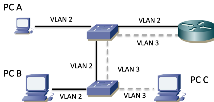
Figura 4 – Topología física con 2 switches
