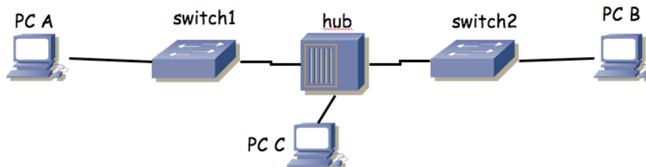
Figura 6- 2 conmutadores interconectados a través de un hub
