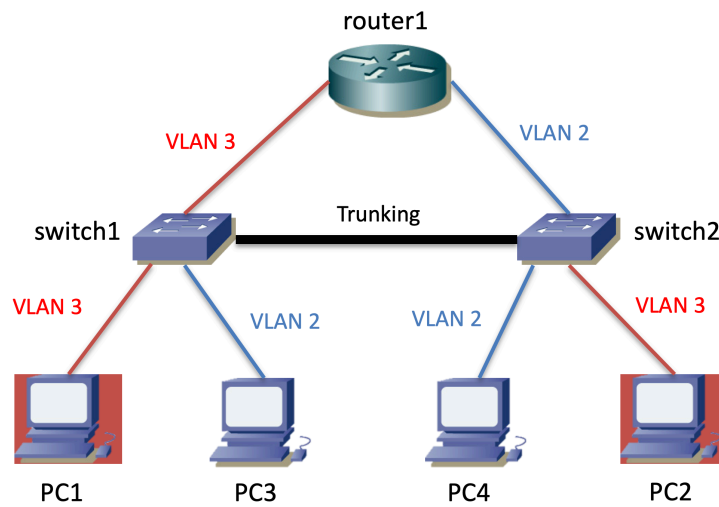
Figura 7- Topología física
