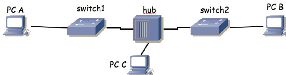
Figura 6- 2 conmutadores interconectados a través de un hub
