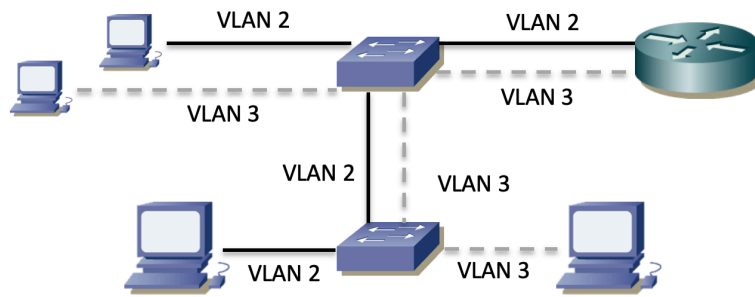
Figura 4- Topología física con 2 switches
