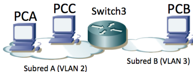
Figura 2 – Topología de capa 3
