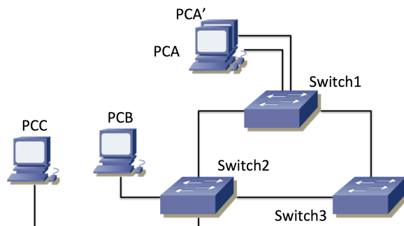
Figura 3 – Topología física con dos interfaces de un PC en uso
