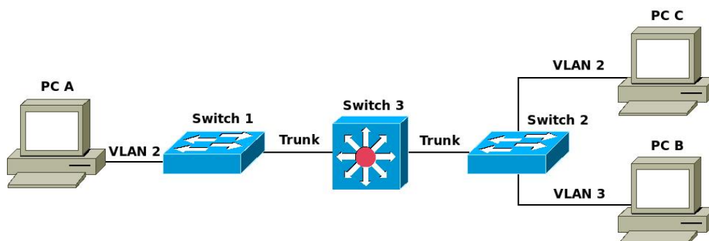
Figura 1.- Dos VLANs encaminadas a través de un conmutador Layer 2/3
