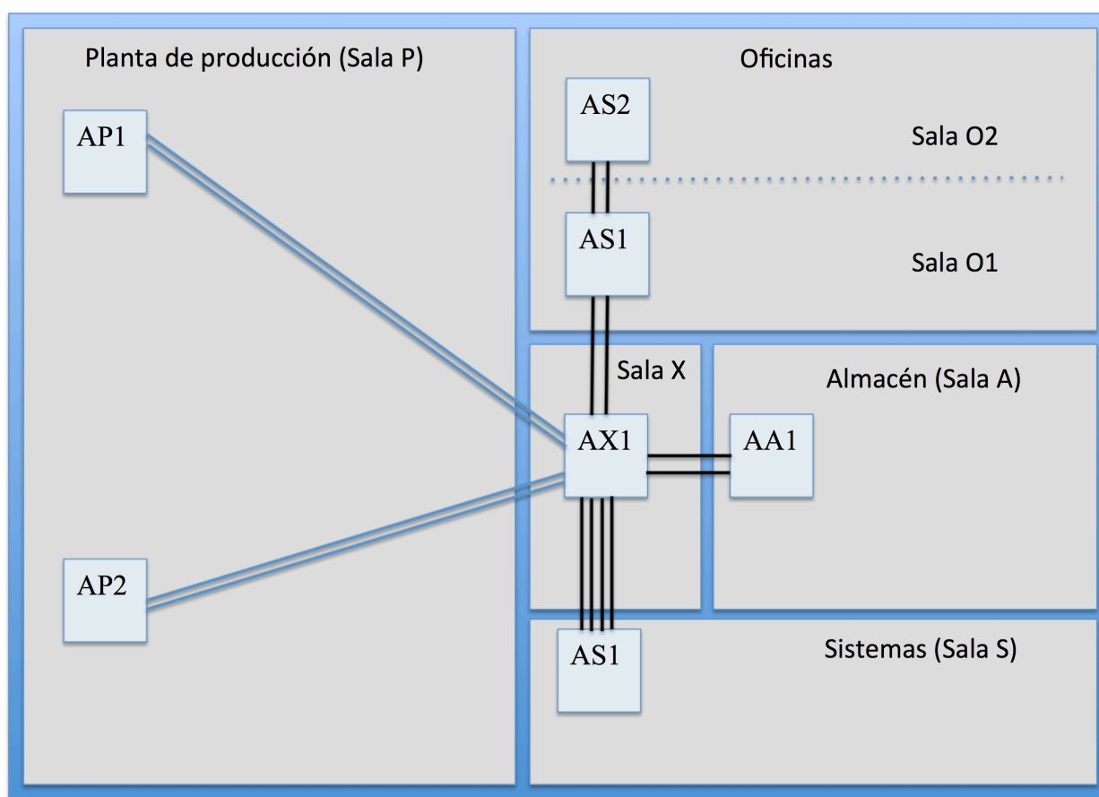
Figura 1 – Esquema de la planta, armarios de comunicaciones y cableado
