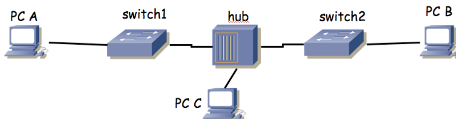
Figura 1.- 2 conmutadores interconectados a través de un hub
