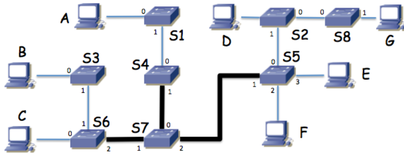
Figura 13 – Topología de red del problema 23
