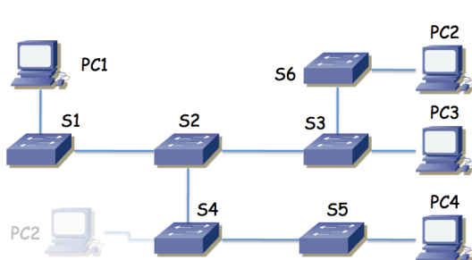
Figura 8.- Topología del problema 9
