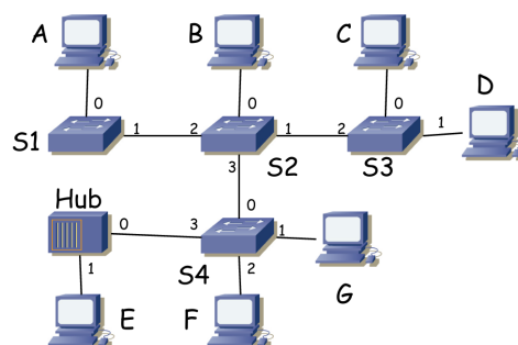
Figura 7.- Topología de la LAN
