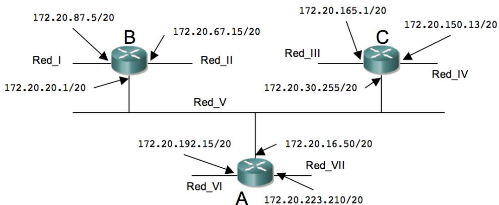
Figura 1.- Topología de la red
