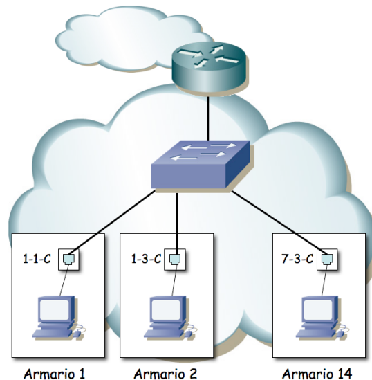
Figura 4.- LAN de prácticas
