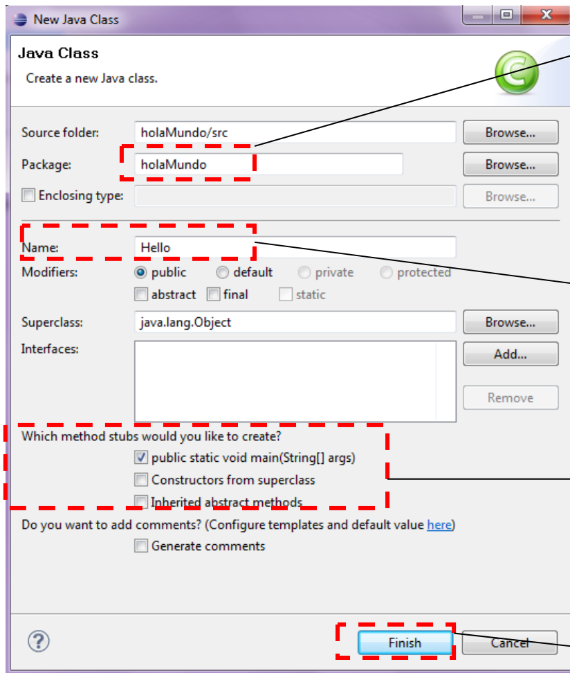
Figura 9: Creación de una nueva clase
