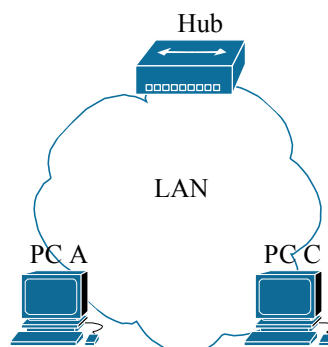
Figura 1. Conexión de 2 PCs en una misma LAN a un hub.
