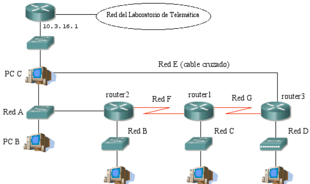
Figura 2.- Routers en línea
