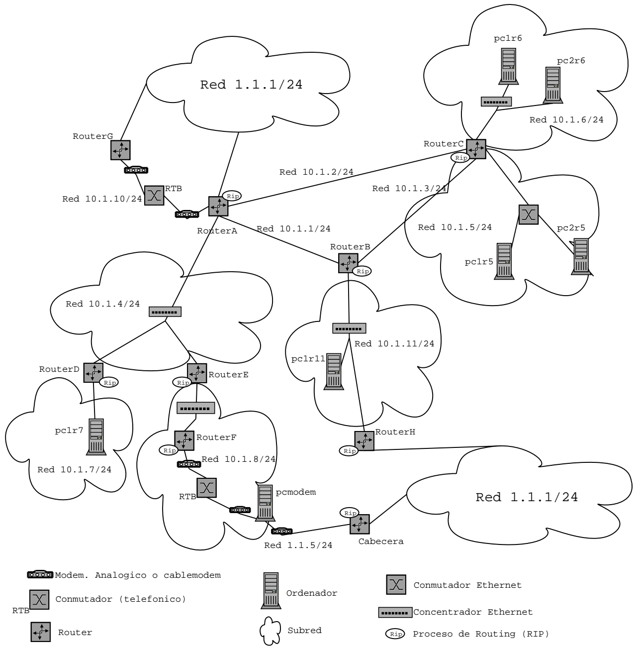
Figura 1: Disposición lógica de las máquinas del laboratorio
